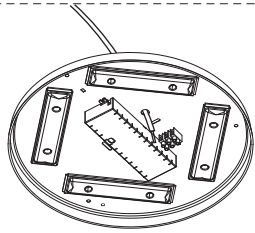
❸ 將輸入線穿過燈具底盤矽膠孔。 Pass the input wire through the hole.
