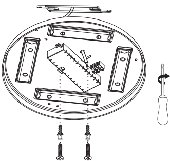
❹ 使用配件包螺絲，將底盤鎖緊在預埋盒上。 Screw the mounting bracket on to the ceiling.
