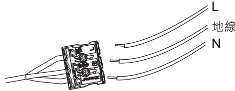
❺ 按壓接線端子，將L、N線與地線按標示接入。 Attach the power wires.
